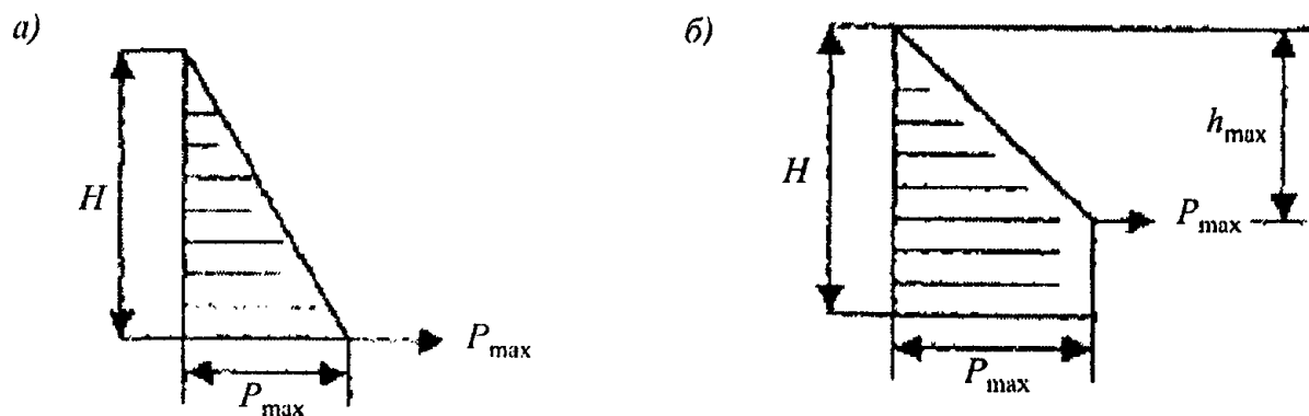
а - гидростатическое давление; б - расчетное давление
