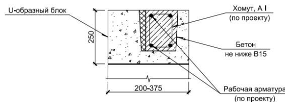
е) Простая U-образная перекрышка
