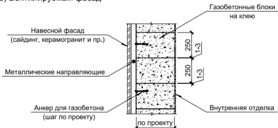
б) Вентилируемый фасад
