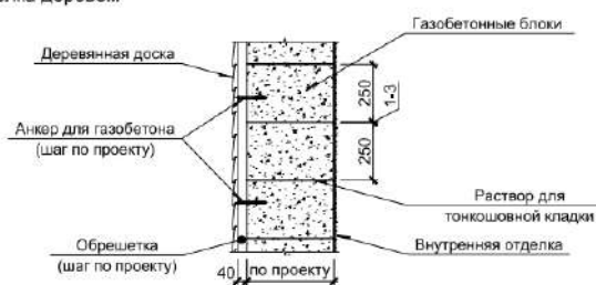
в) Отделка деревом
