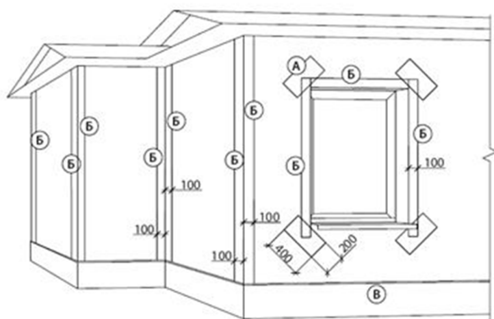
Рис. 17. Схема армирования штукатурки: А — углы проемов. Сетка 200×400 мм; Б — углы кладки, ребра откосов. Угловой профиль и сетка. Нахлест сетки по 100 мм. Ширина полотна 100 + 100 = 200 мм; В — примыкание к цоколю. Цокольный стартовый профиль.
