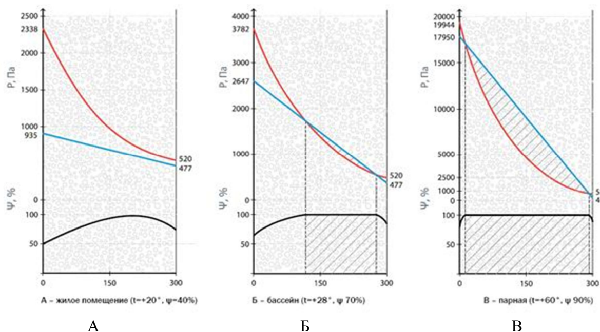
Рис. 26. Влияние микроклимата на распределение влажности воздуха в порах по толщине стены: А – жилое помещение ( t = 20^{\circ} , \psi = 40\% ); Б – бассейн ( t = 28^{\circ} , \psi = 70\% ); В – баня ( t = 60^{\circ} , \psi = 90\% ).
