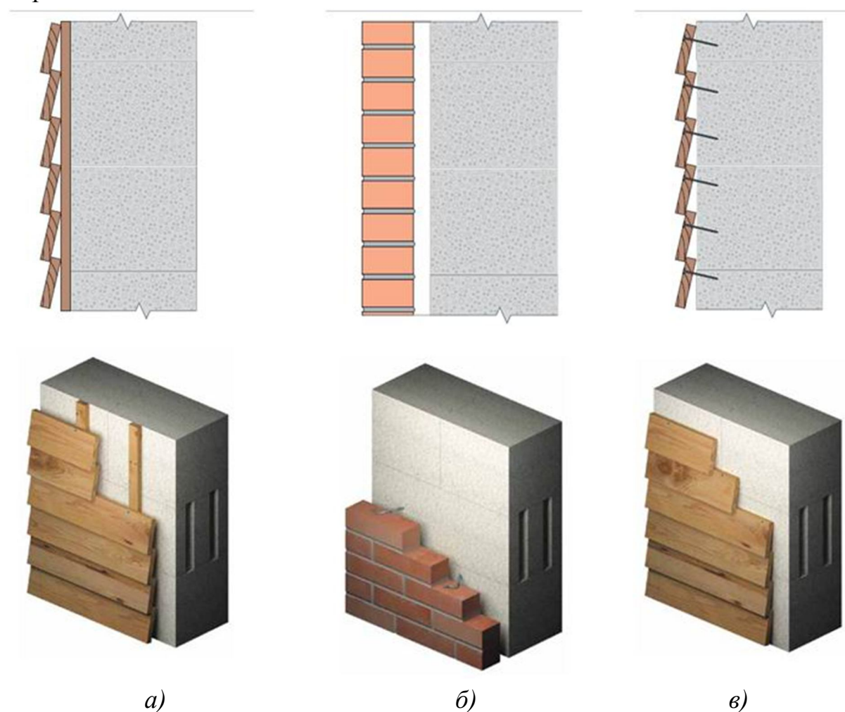
Рис. 9. Облицовка на отnose: а — крепление облицовочных изделий к направляющим; б — облицовка кладкой из штучных материалов; в — механическое крепление штучных материалов к кладке
