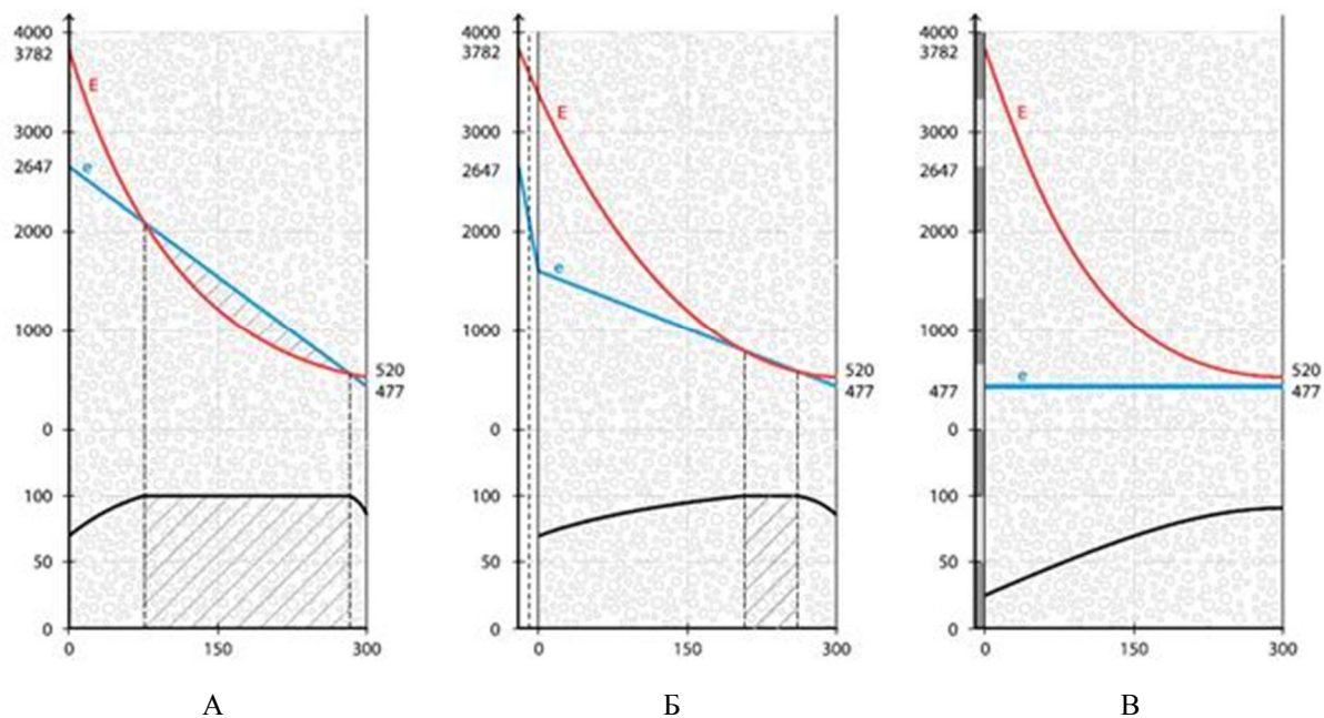
Рис. 28. Влияние внутренней пароизоляции на распределение влажности воздуха в порах по толщине стены: А — без внутренней отделки; Б — слой цементно-песчаной штукатурки; В — паронепроницаемая отделка.
