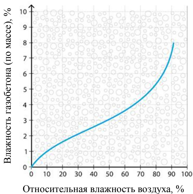
Рис. 7. Обобщенная изотерма сорбции газобетона
