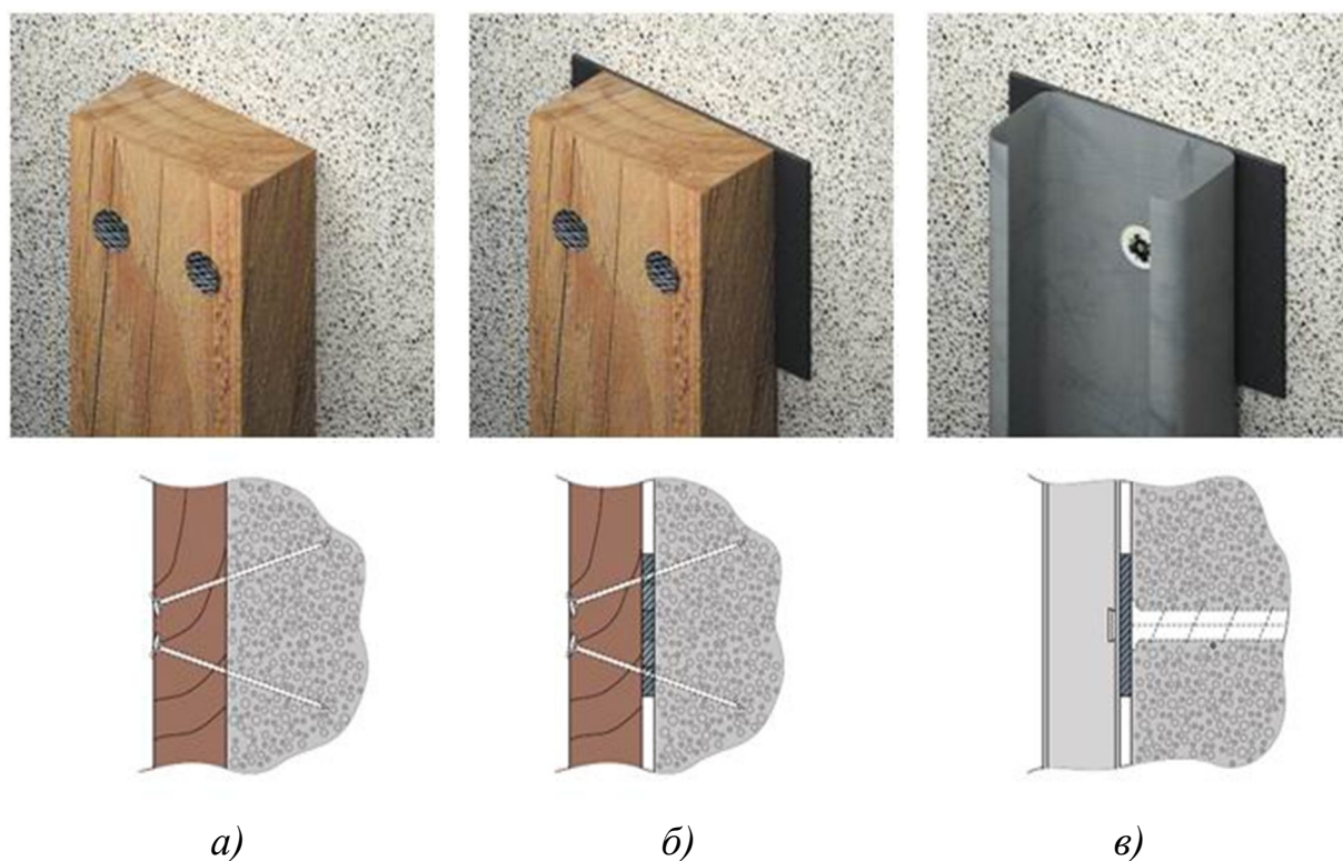
Рис. 11. Установка направляющих: а — деревянная обрешетка по подсохшей кладке; б — деревянная обрешетка по влажной кладке; в — металлическая обрешетка
