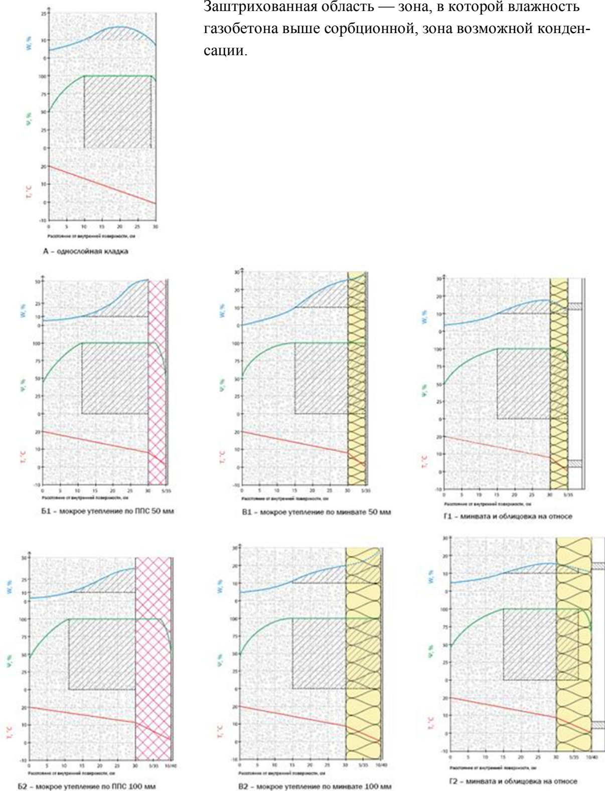
Рис. 23. Распределение влаги, температуры и влажности воздуха в порах материала по толщине стены в первый отопительный сезон.
