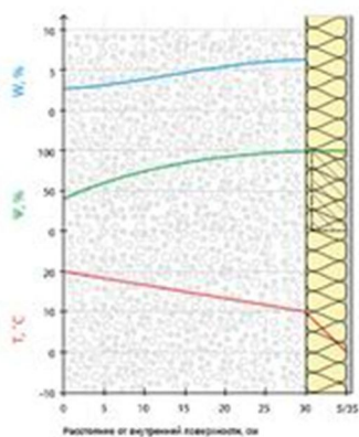
В1 – мокрое утепление по минвате 50/
