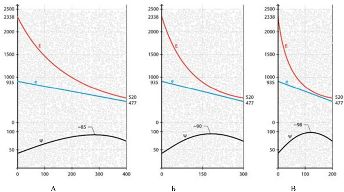
Рис. 27. Влияние толщины конструкции на распределение влажности воздуха в порах по толщине стены: А — 400 мм; Б — 300 мм; В — 200 мм
