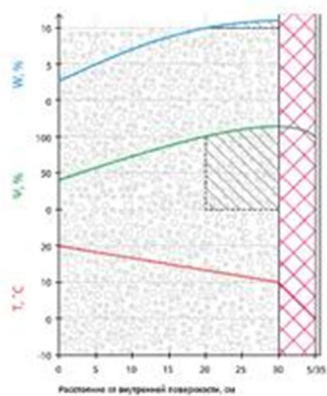
Б1 – мокрое утепление по ППС 50/100 мм
