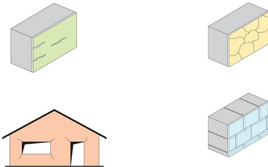
Рис. 19. Основные типы дефектов штукатурки
