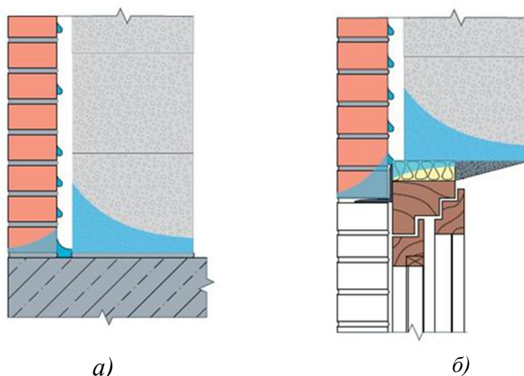
Рис. 10. Конденсат на внутренней поверхности облицовок.
