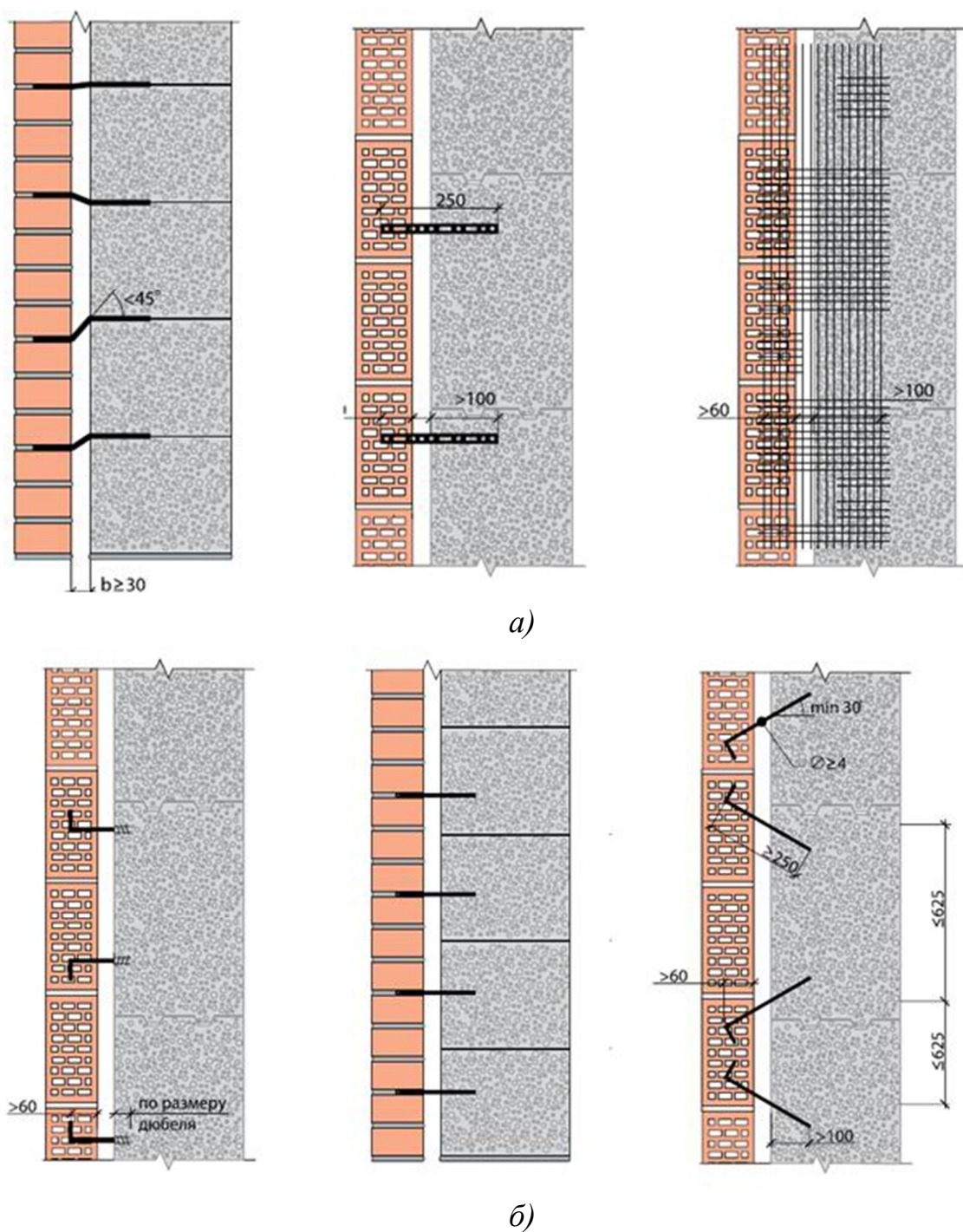
Рис. 16. Связь облицовочного и основного слоев кладки:
