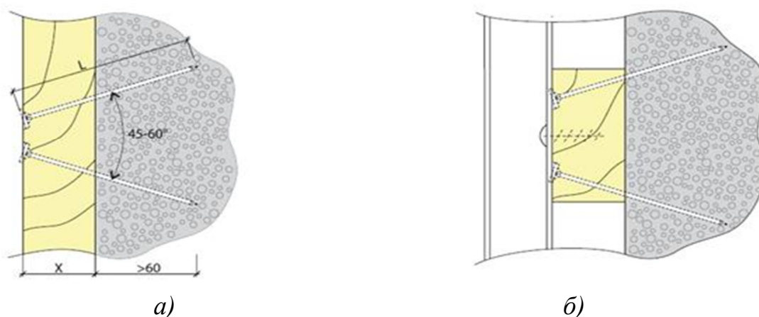
Рис. 12. Гвоздевое крепление обрешетки: а — деревянный брусок, набитый на кладку непосредственно; б — крепление профиля через опорный брусок
