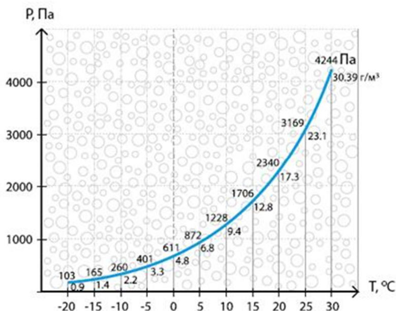
Рис. 25. Давление насыщения водяного пара и максимальное влагосодержание воздуха в зависимости от температуры
