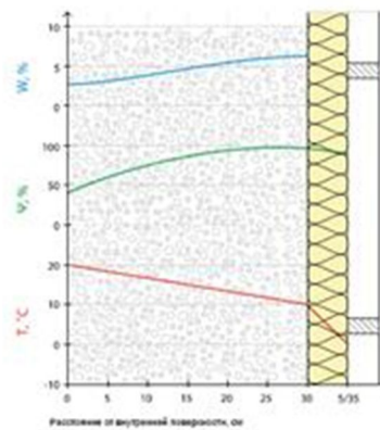
Г1 – минвата и облицовка на отnose
