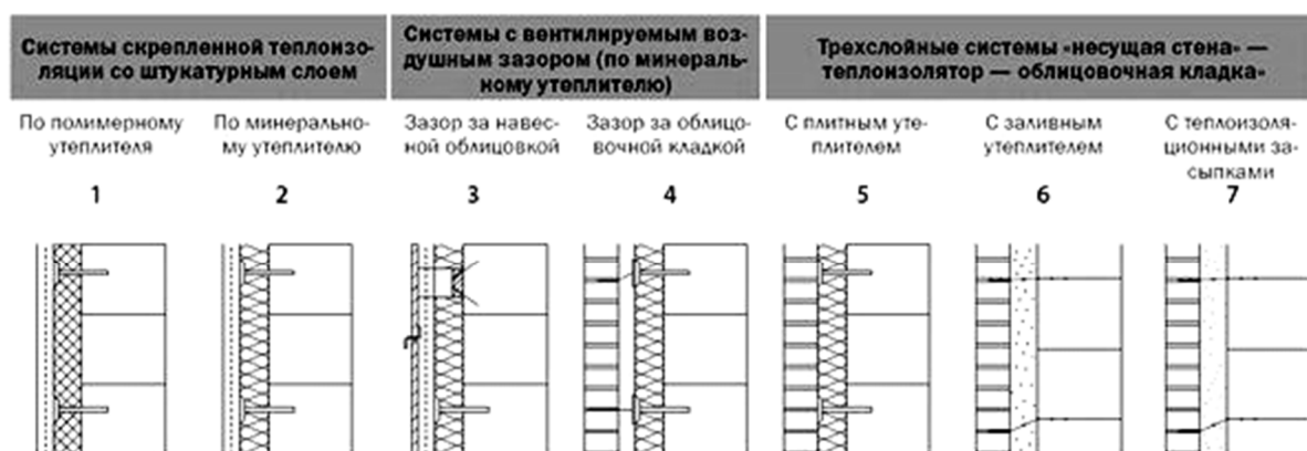
Рис. 20. Системы теплоизоляции
