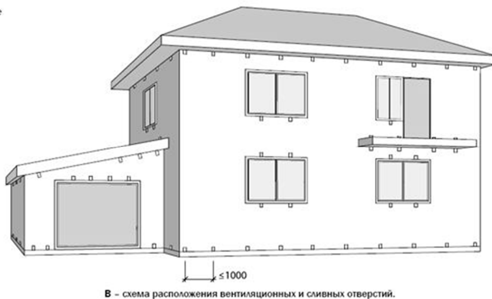
Рис. 14. Меры по отводу конденсата из зоны потенциального увлажнения
