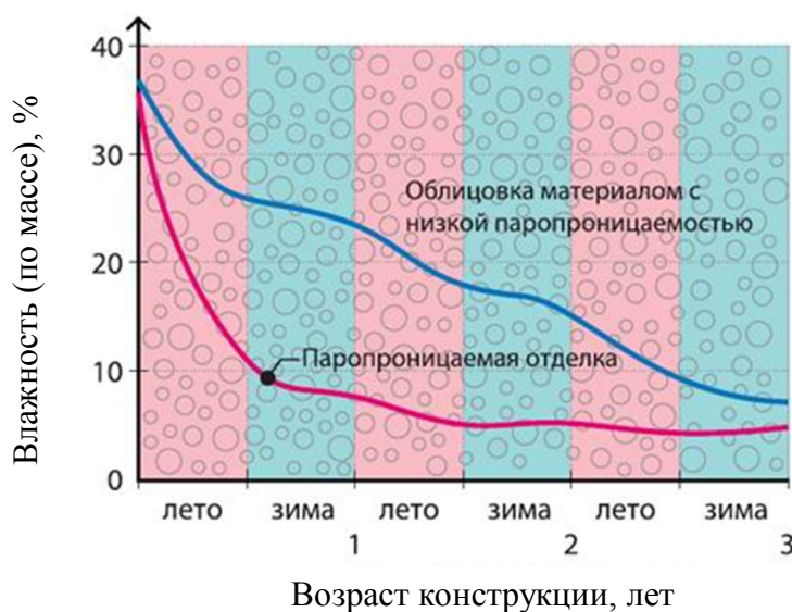
Рис. 8. Высыхание газобетона в однослойных конструкциях
