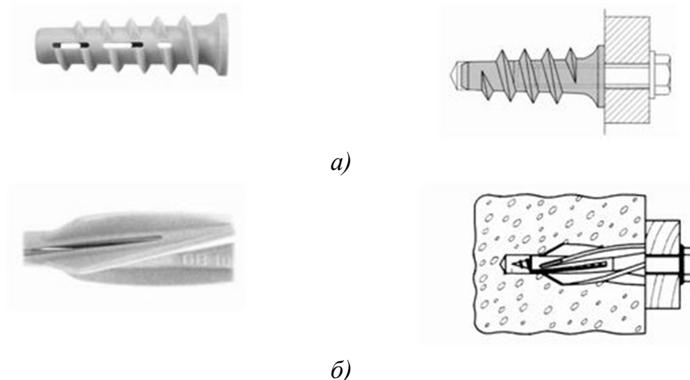
Рис. 13. Фотографии и схемы из каталога «Фишер. Крепежные системы»: а — Фишер ФТП, Сормат КБТ; б — Фишер ГБ
